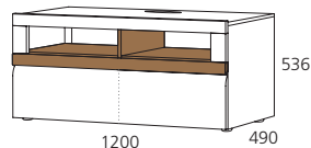
PZ-TV421G (1 DVOJNI PREDAL / DUPLA LADICA / DOUBLE DRAWER, 1 KLOPNA VRATA / POKLOPNA VRATA / FLAP DOOR)
