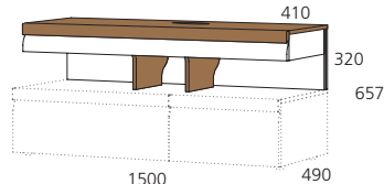
PZ-TVN5 (1 KLOPNA VRATA / POKLOPNA VRATA / FLAP DOOR)
