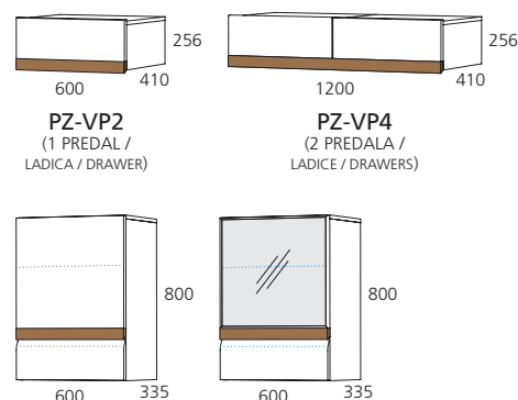
PZ-VL21 L PZ-VL21 D (1 VRATA / VRATA / DOOR)
