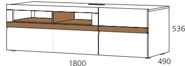
PZ-TV621G (L, D) (2 PREDALA / LADICE / DRAWERS, 1 DVOJNI PREDAL / DUPLA LADICA / DOUBLE DRAWER, 1 KLOPNA VRATA / POKLOPNA VRATA / FLAP DOOR)
