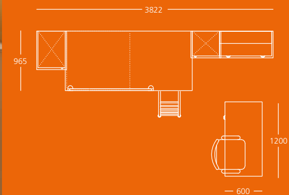
detajl tx-1b
