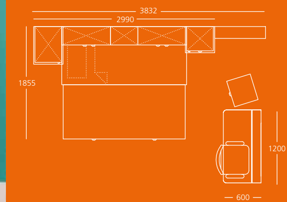
detajl tx-2b
