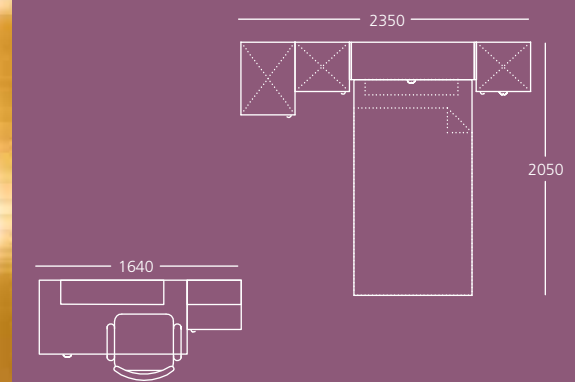
detajl ty-4b
